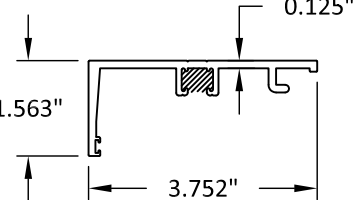
⑦ 3 1/4" SUBFRAME
