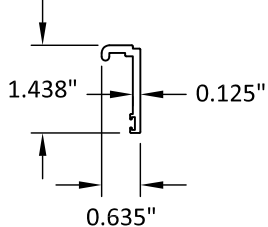
⑪ T-MULLION
